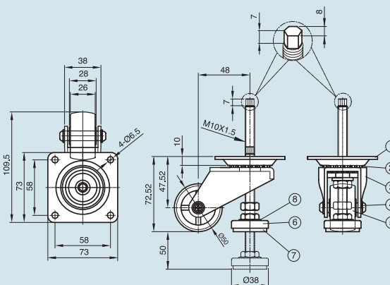
APLC-200 Type
